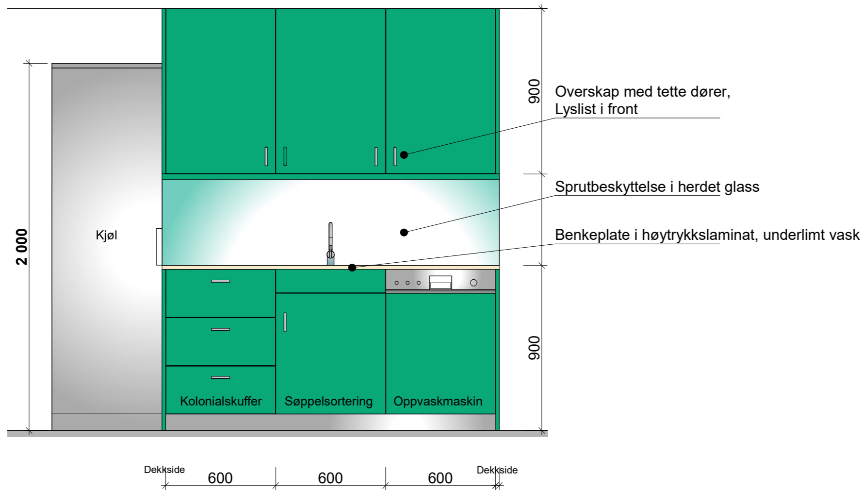
Oppriss C
